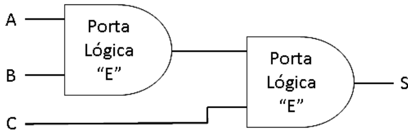
Figura 2. Conectando várias portas lógicas "E".
