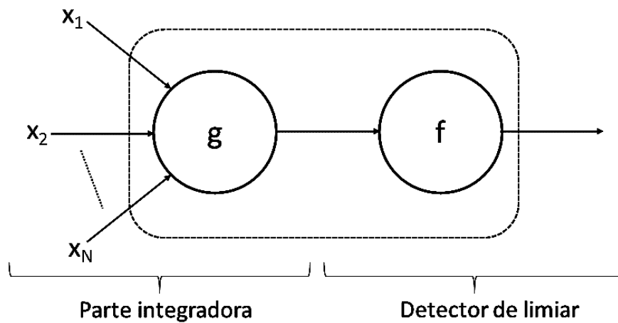
Figura 1. Modelo simplificado de neurônio proposto por Warren McCulloch e Walter Pitts. ROJAS, 1996 (com adaptações).
