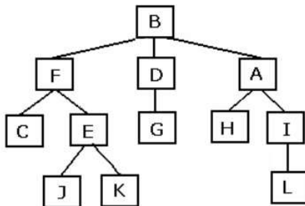
Figura 1. Busca em profundidade. RUSSELL e NORVIG, 2004.
