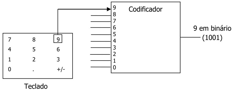
Figura 2. Codificador. THOMAS, 2007.
