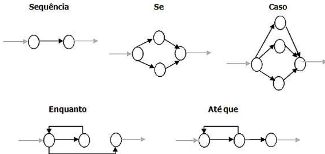
Figura 1. Notação de um grafo de fluxo. Pressman (2002).
