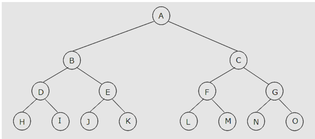
Figura 2. Árvore binária completa. Salvetti, 1993.
