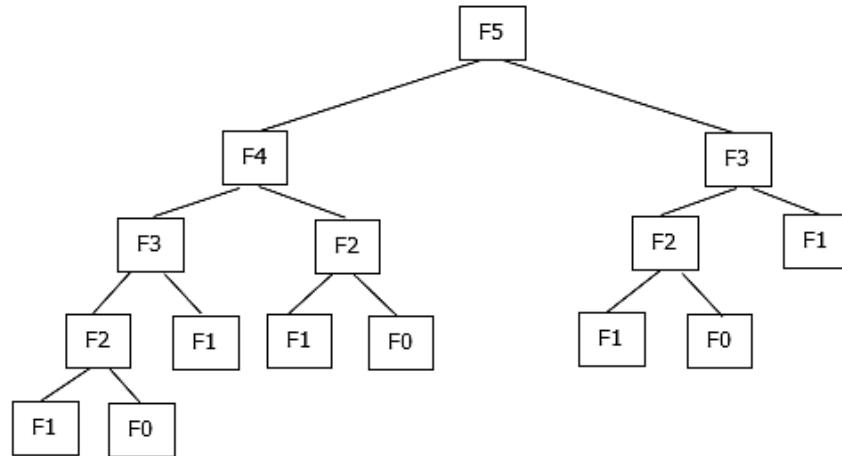
Figura 1. Ocorrências da função \text{fib}(n) .
