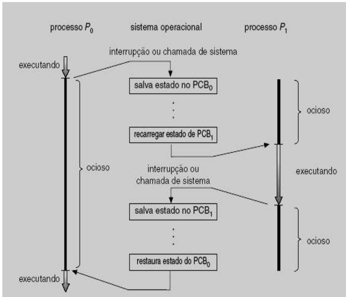
Figura 1. Troca de um processo que está sendo executado pela CPU por outro. Silberschatz, Galvin e Gagne, 2008.
