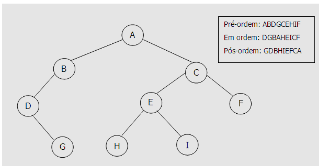
Figura 3. Percorrendo uma árvore em pré-ordem, em ordem e pós-ordem. Tenenbaum, 1995.
