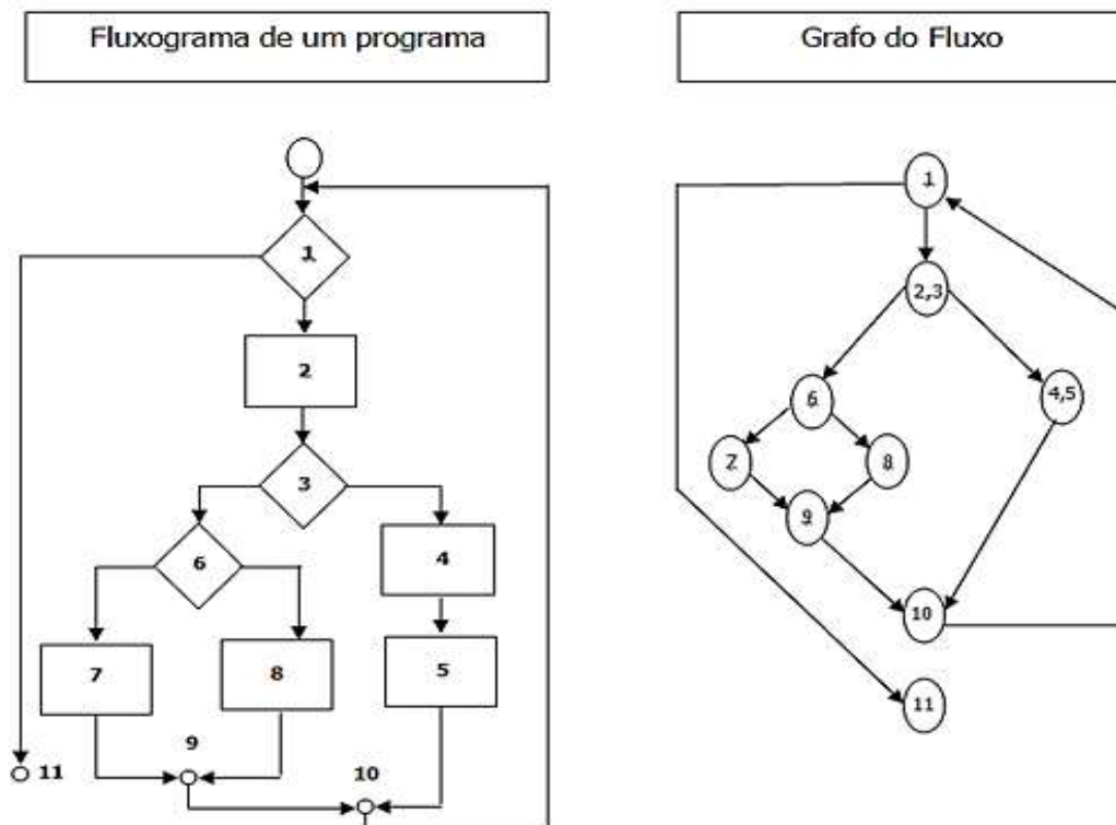
Figura 2. Mapeamento de um fluxograma em um grafo de fluxo. Pressman (2002).
