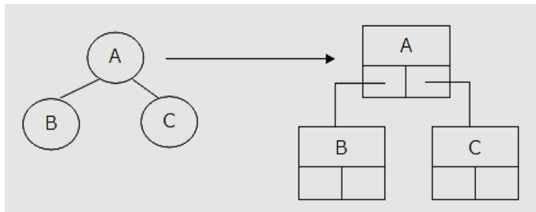
Figura 4. Árvore binária na qual seus registros estão subdivididos em três elementos (chave, esquerdo e direito).
