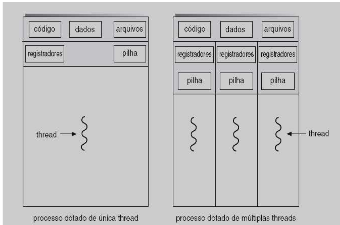
Figura 2. Detalhamento de uma thread. Silberschatz, Galvin e Gagne, 2008.
