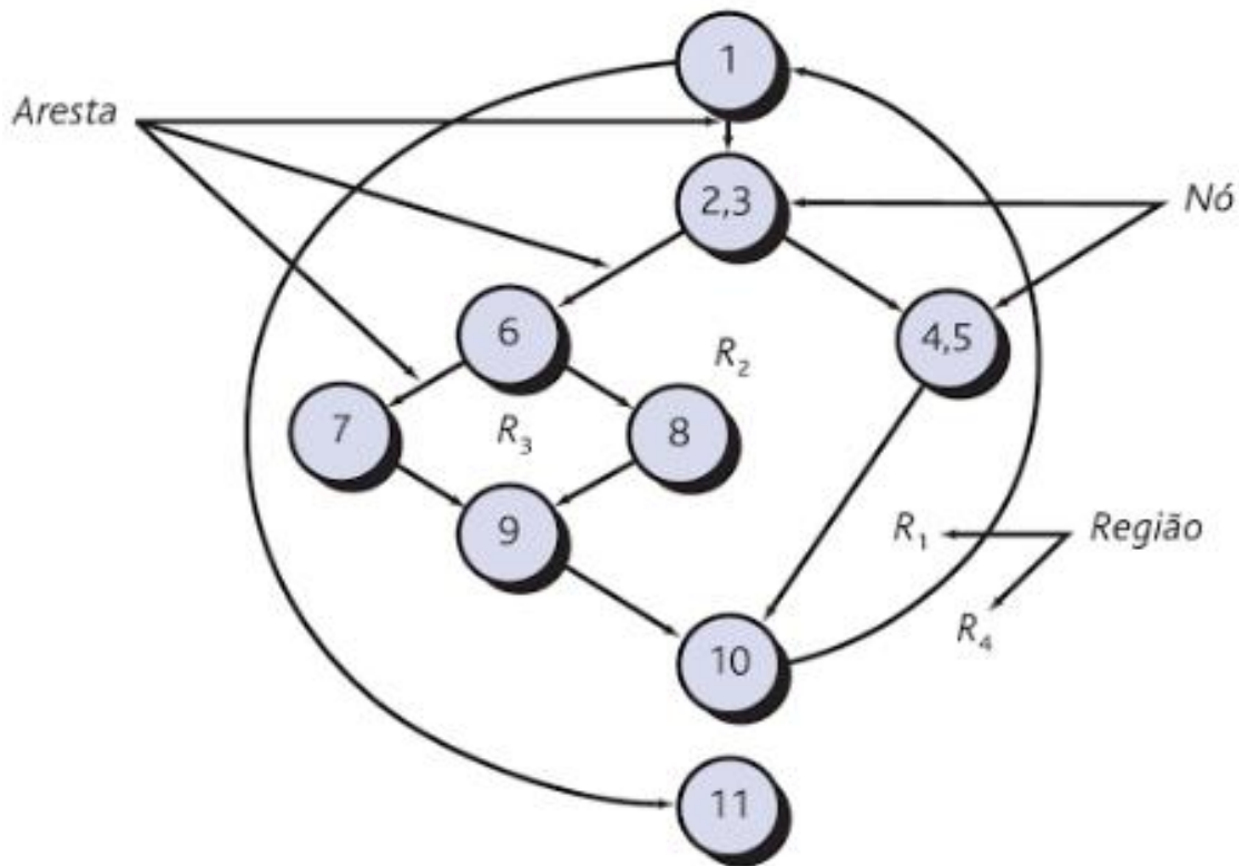
Figura 2. Exemplo de fluxograma da estrutura de um programa. PRESSMAN, R. S; MAXIM, B. R. (2021).
